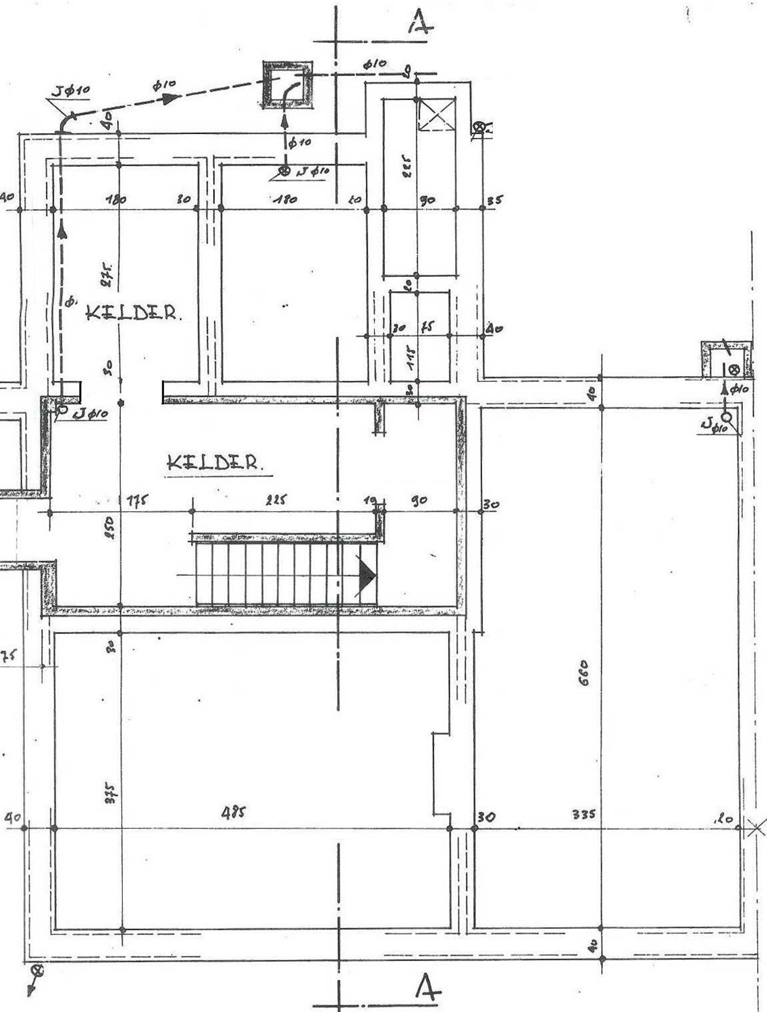
FUNDIERUNGSPLAN
